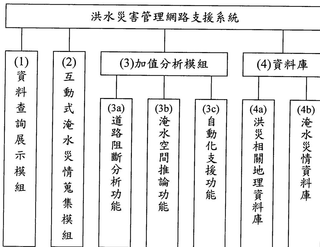
圖 3-1 洪水災害管理網路支援系統架構圖
