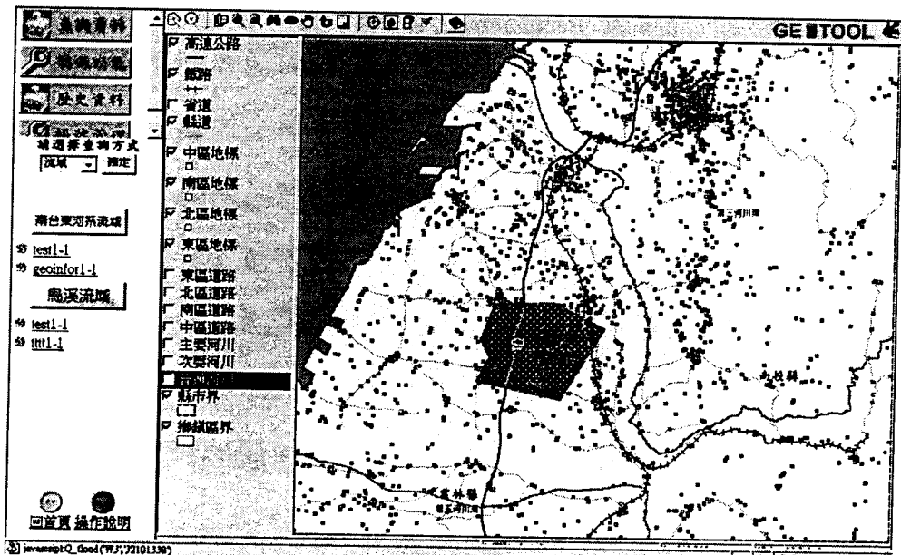
圖 2-18 經濟部水利處 GIS 應用測試中心淹水查詢系統 ( http://210.69.128.6/flood/home.htm )
