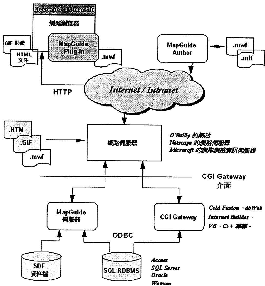
圖 2-3 MapGuide 解決方案架構圖 (九福科技, 2000)
