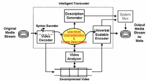
圖 7：通用可擴充性壓縮之壓縮系統之方塊圖。
