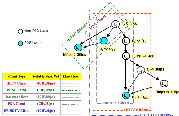
圖 3：實做系統中的視訊擴充結構圖。
