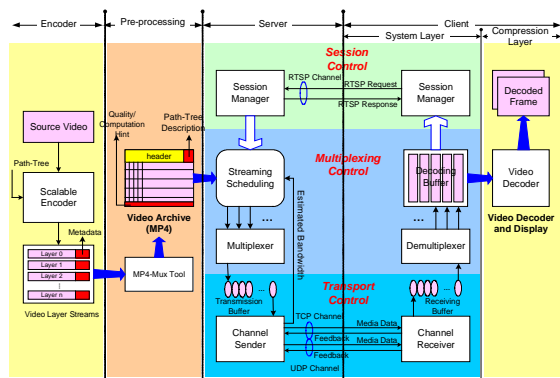
圖 9：通用可擴充性壓縮之串流伺服器與內容資料產生與消耗之流程示意圖。
