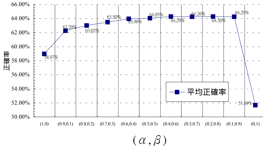
圖 3 語意與詞類比重( \alpha, \beta )與正確率關係圖
