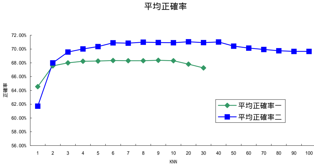
圖 5 相似詞數量(KNN)與正確率關係
