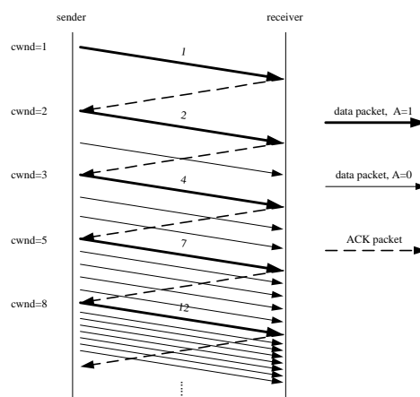
圖一、 Congestion window growth
