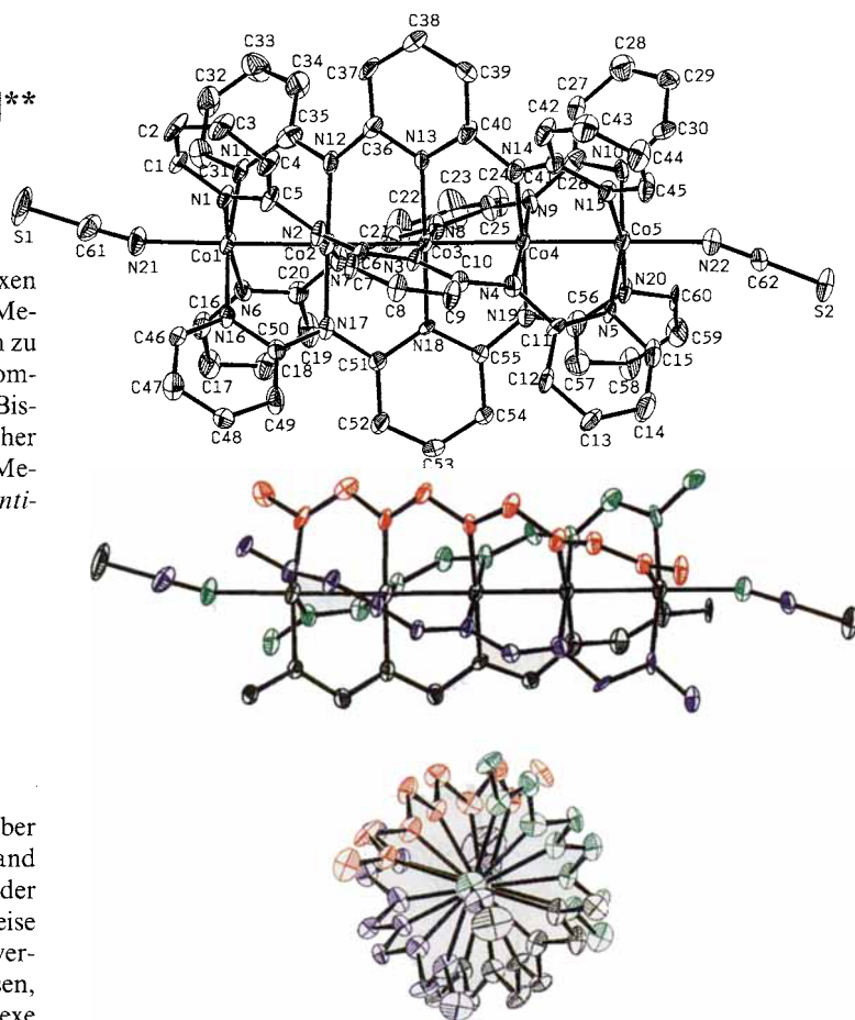
Abb. 1. Oben: Struktur von [\text{Co}_5(\mu_5\text{-tpda})_4(\text{NCS})_2] im Kristall. Ausgewählte Bindungslängen [Å] und -winkel [°]: Co1-Co2 2.277(2), Co2-Co3 2.232(2), Co3-Co4 2.229(2), Co4-Co5 2.274(2), Co1-N21 2.07(1), Co1-N(py) (Durchschnittswert) 1.97(1), Co2-N (Durchschnittswert) 1.90(1), Co3-N (Durchschnittswert) 1.93(1), Co4-N (Durchschnittswert) 1.90(1), Co5-N(py) (Durchschnittswert) 1.97(1), Co5-N22 2.06(1); N21-Co1-Co2 178.8(3), Co1-Co2-Co3 178.7(1), Co2-Co3-Co4 179.9(1), Co3-Co4-Co5 178.8(1), Co4-Co5-N22 179.3(3), N(py)-Co1-Co2 (Durchschnittswert) 86(1), N-Co2-Co3 (Durchschnittswert) 89(1), N-Co3-Co4 (Durchschnittswert) 90(1), N-Co4-Co3 (Durchschnittswert) 89(1), N(py)-Co5-Co4 (Durchschnittswert) 86(1). Mitte: Darstellung der helicalen Anordnung der Liganden an der linearen Metallkette (nahezu senkrecht zur Metallkette). Die drei Kohlenstoffatome der Pyridinringe sind aus Gründen der Übersichtlichkeit weggelassen. Unten: Ansicht entlang der Metallkette.
