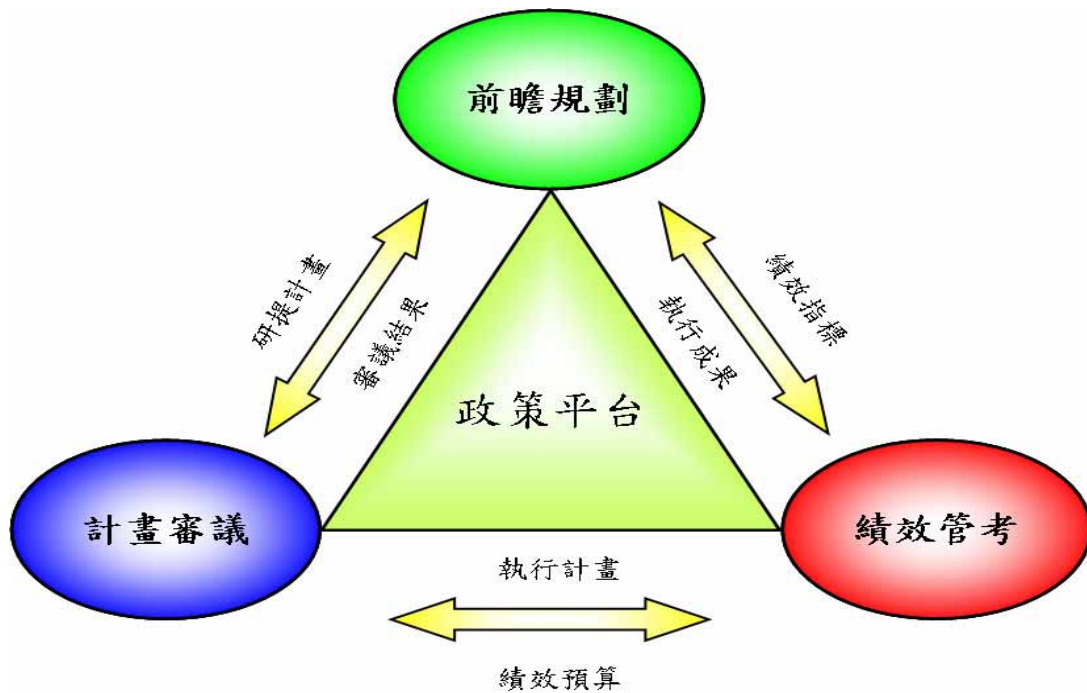
圖一 科技計畫規劃、審議與管考一貫化及相互扣連關係圖
