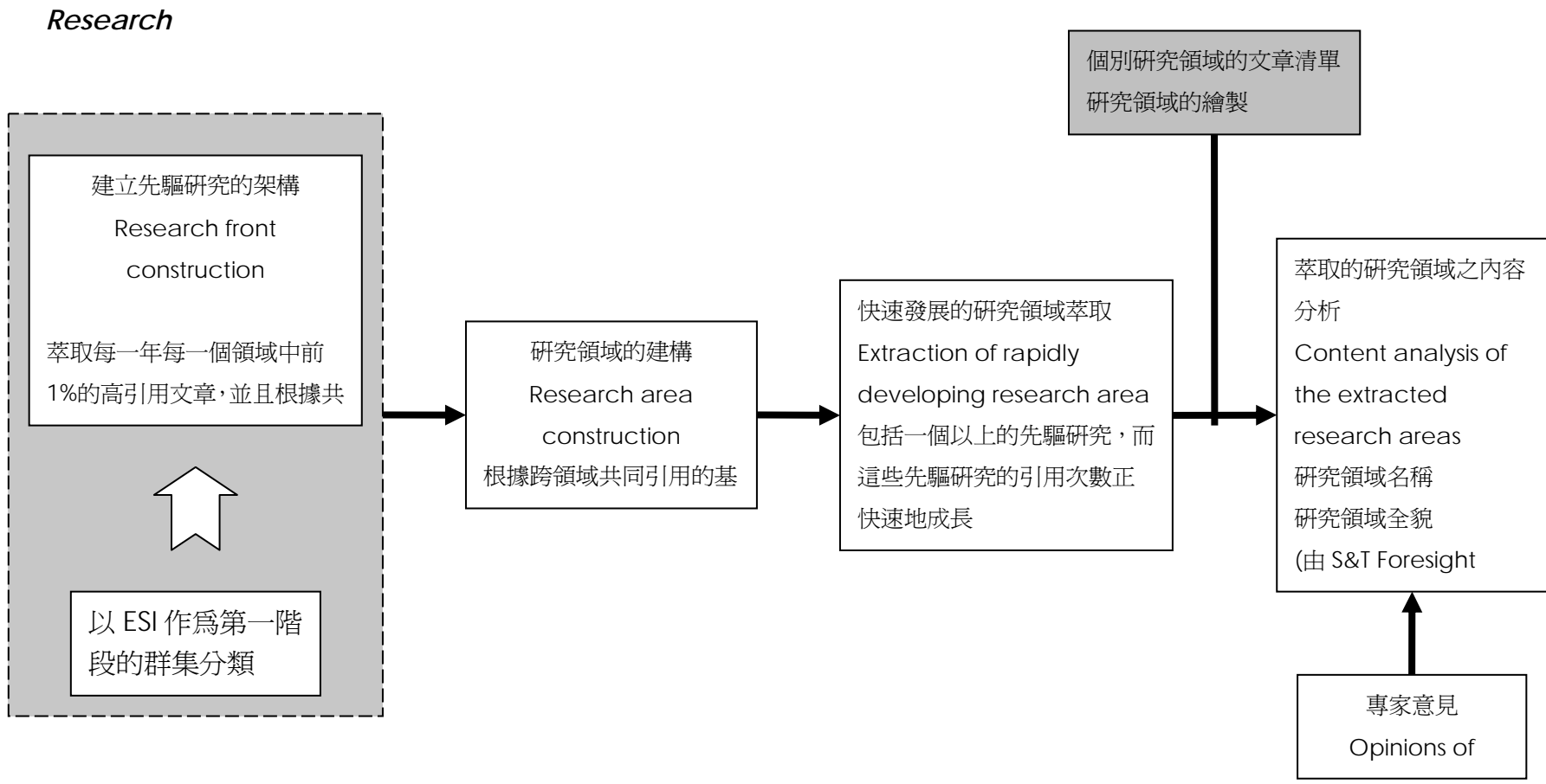
圖九 快速發展的研究領域調查研究流程圖
