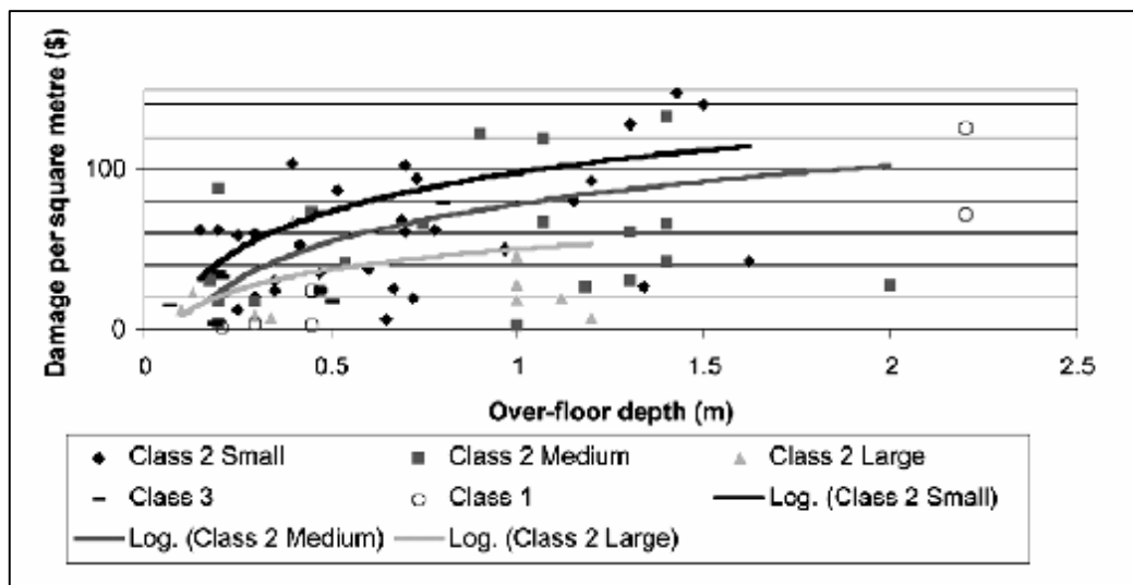
圖 4-20. Kempsey 淹水資料分群平均迴歸圖
