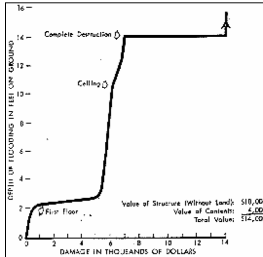
圖 4-4. FEMA 一層無地下室住宅淹水深度-損失曲線
