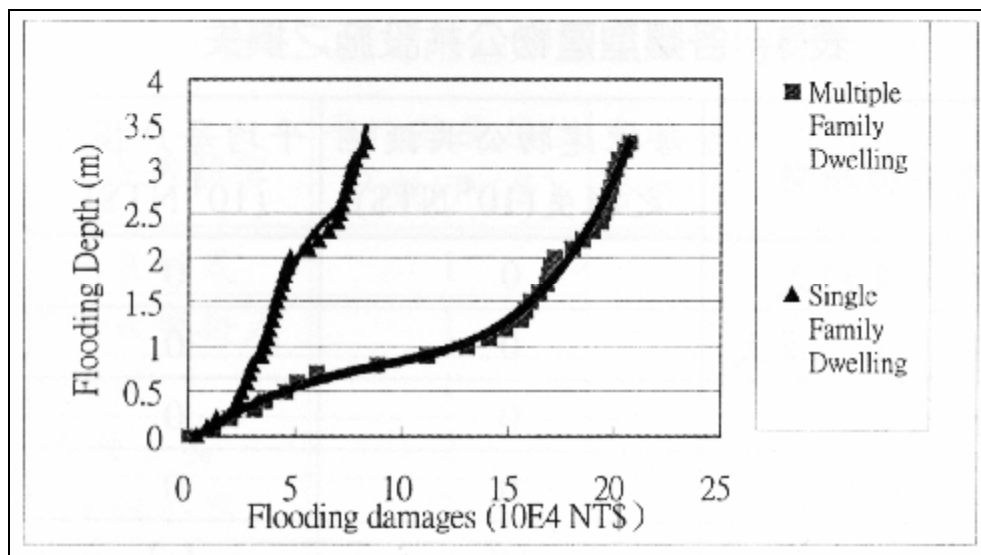
圖 4-7. 集合住宅與單一住宅淹水深度-損失曲線
