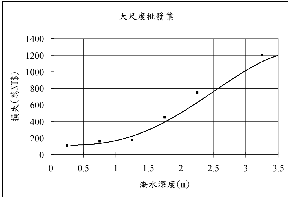
圖 4-12. 大尺度批發業淹水深度-損失曲線
