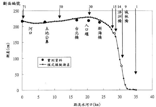
圖 7 實測資料與模式模擬之潮差比較(銜接點為浮洲橋)
