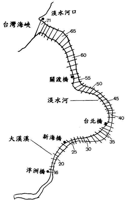
圖 4 淡水河-大漢溪平面圖及各河段編號(以浮洲橋為銜接點)
