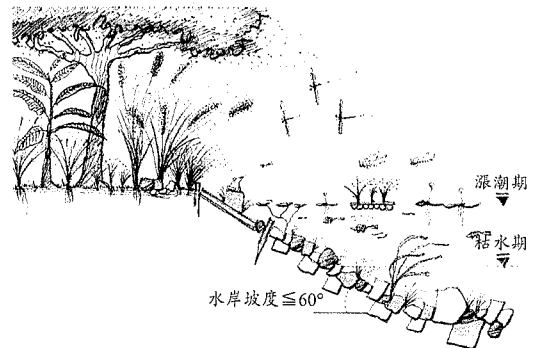
圖 12 綜合式水岸設計圖例(以保育類褐樹蛙需求為例)
