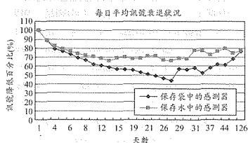
圖 4.3 感測器保存在密封袋與密閉水中訊號衰退的情況
