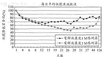
圖 4.5 感測器的電解液濃度對老化的影響
