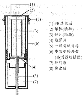
圖 3.1 自製溶氧感測器示意圖
