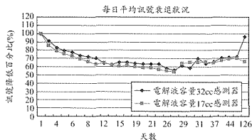
圖 4.6 感測器的電解液容量對老化的影響
