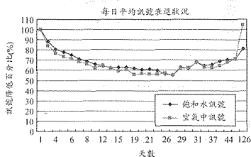
圖 4.2 感測器在飽和溶氧水與空氣中訊號衰退的情形
