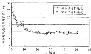
圖 4.4 自製溶氧感測器每日訊號老化速度關係圖
