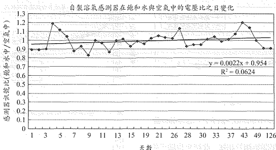
圖 4.1 感測器在飽和溶氧水與空氣中的電壓比之日變化
