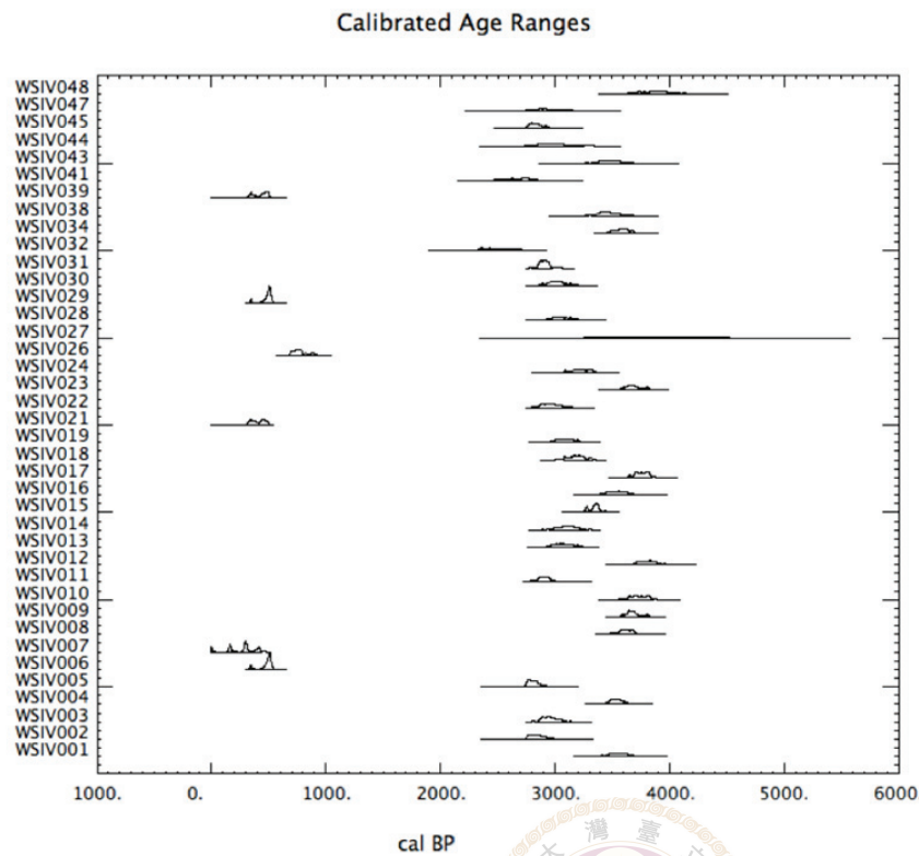
圖 2 碳十四年代校正圖
