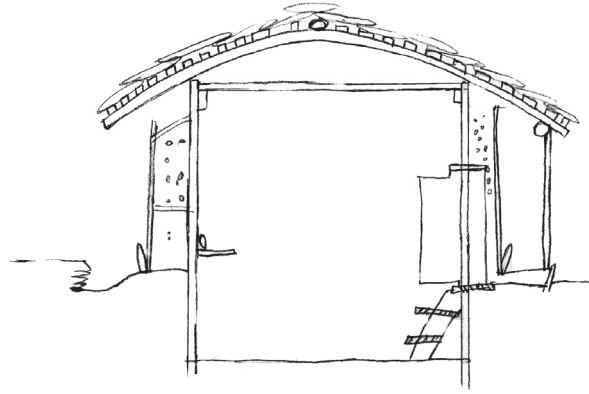
圖 12 於屋內入口處採用木梯之豎穴式建築
