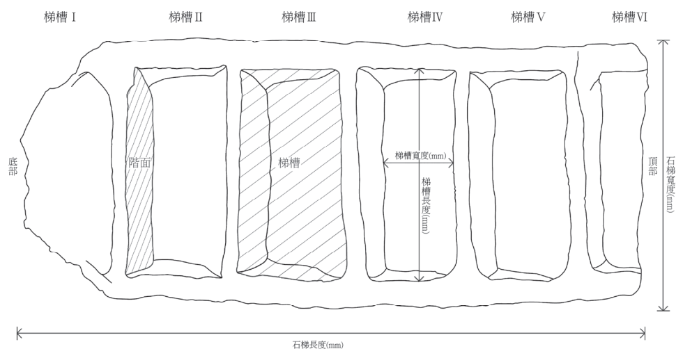
圖 1 「石梯」俯視圖繪測成果及記錄屬性說明（以 PNSL001 為例，劉宜婷繪）
