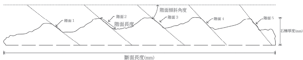
圖 2 「石梯」剖面俯視圖繪測成果及階面傾斜角之量測說明（以 PNSL001 為例，劉宜婷繪）
