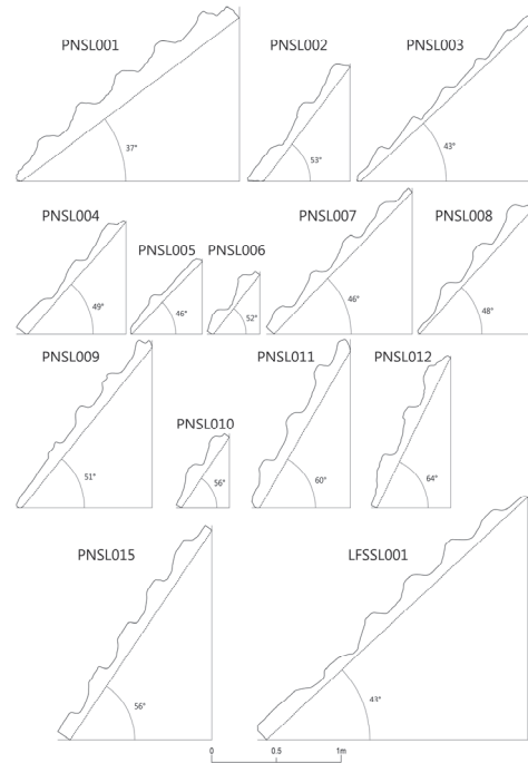
圖 7 「石梯」以最小階面傾斜角度模擬使用之情形(劉宜婷繪)
