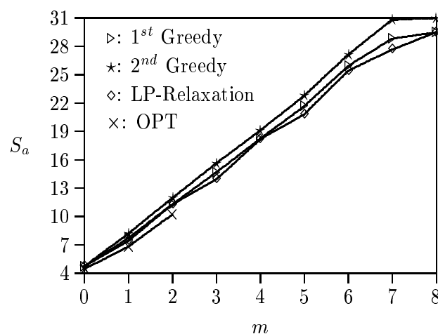
(d) Hudson's data (40 SNPs)
