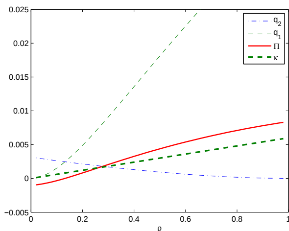
圖 2: 淨利率 a < 0 的均衡
