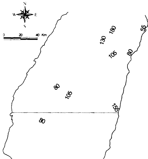
圖一：台灣中部地表二氧化矽熱流量分布圖。
