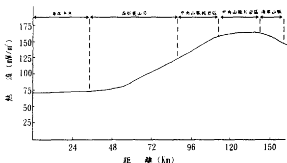
圖二：台灣中部地表二氧化矽熱流量東西向剖面分布圖。
