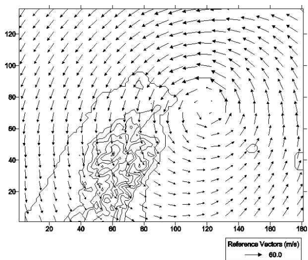
圖七 雷達解析颱風渦旋植入 MM5 模式模擬賀伯颱風 19960731_06:00 之初始場的 850 mb 水平風場
