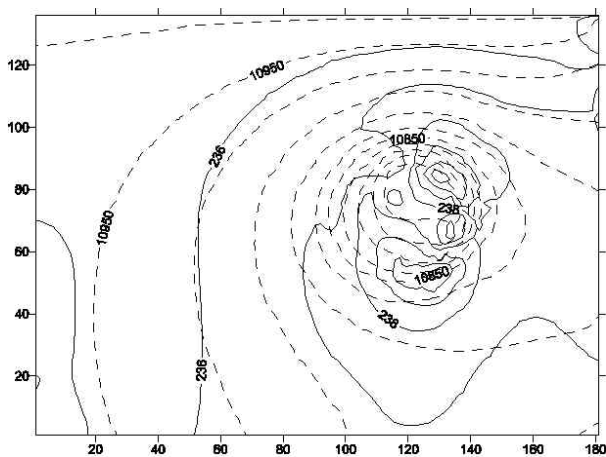
圖十二 同圖十之 250 mb 平衡質量場
