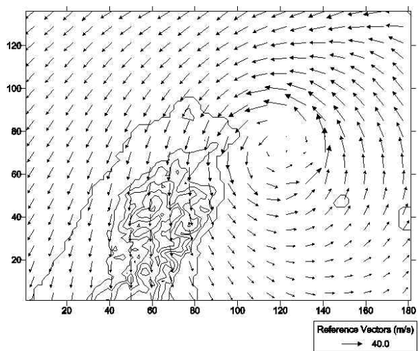
圖九 同圖七之 250 mb 水平風場
