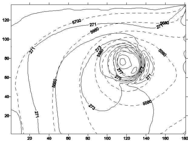
圖十一 同圖十之 500 mb 平衡質量場
