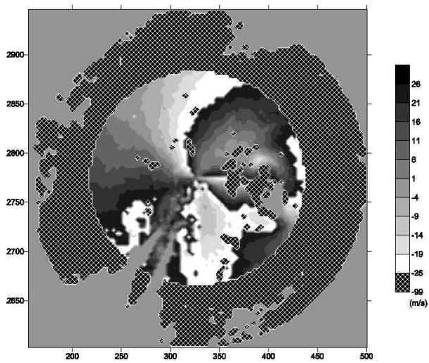
圖一 1996 年 7 月 31 日 11:02 五分山雷達最低仰角 (0.48 度) 之原始都卜勒風場觀測資料 (m/s)
