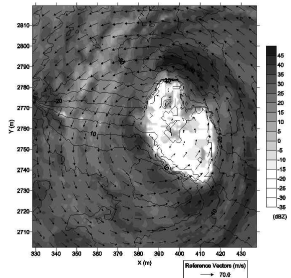
圖六 利用 GBVTD 法解析 19960731_11:02 兩公里高的颱風渦旋水平風場(箭號)。圖中等值圖為雷達回波圖，等值線為雷達都卜勒風速觀測。
