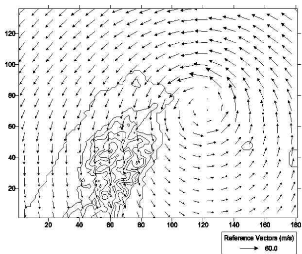
圖八 同圖七之 500 mb 水平風場
