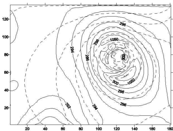
圖十 與圖七 850 mb 之水平風場平衡的質量場，實線為等溫線(K)，虛線為等高線(m)
