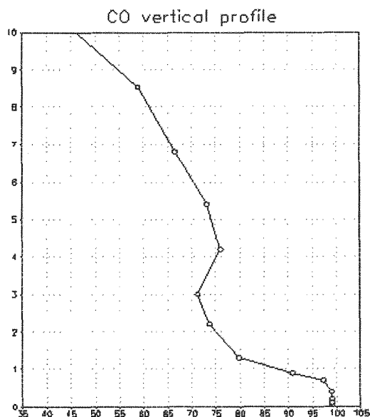
圖 9 模擬之蘭嶼近地面臭氧與實測資料比較，及模擬之蘭嶼上空 CO 垂直剖面。
