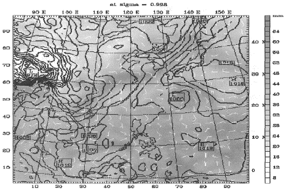
(a)1996/7/16 12Z
