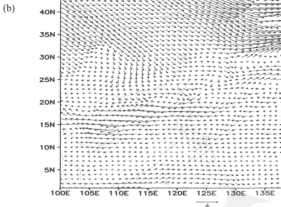
圖 4 1996 年(a)7 月 17 日 02Z 與(b)12 月 20 日 02Z，模擬得在 850hPa 水平臭氧通量 ( 10^{-9} moles \text{cm}^{-2} \text{s}^{-1} ) 分布圖。
