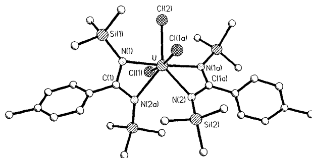
Abb. 1. Struktur von 1 im Kristall [6, 7]. Ausgewählte Bindungslängen [pm] und -winkel [°]: U-Cl(1) 256.8(5), U-Cl(2) 252.7(5), U-N(1) 226.5(8), U-N(2) 237.2(5), C(1)-N(2) 132.3(11), C(1)-N(2a) 131.9(11); N(1)-U-N(2a) 57.5(2), N(1)-U-N(1a) 176.4(3), N(1)-C(1)-N(2a) 115.3(6), Cl(1)-U-Cl(1a) 170.7(2).
