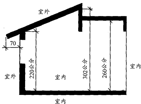
圖 2 實驗空間剖面圖
